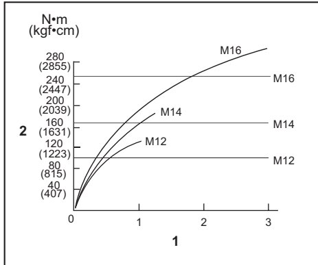
1. Tilspændingstid (sekunder) 2. Tilspændingsmoment
