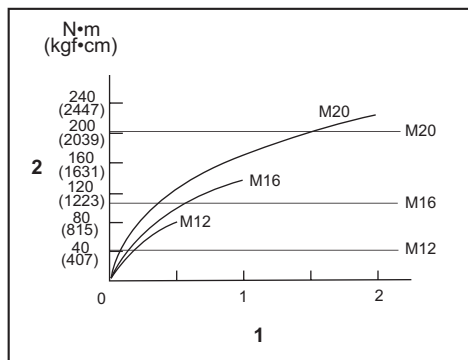
1. Χρόνος στερέωσης (δευτερόλεπτο) 2. Ροπή στερέωσης
